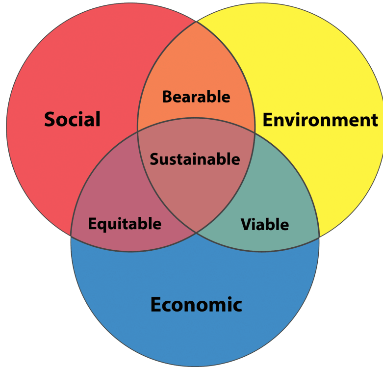
Venn diagram
